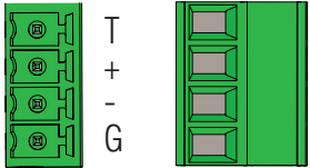
RS-485 P3-RS485CON-1
